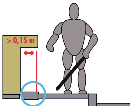
Surépaisseur détectable 3 cm minimum
