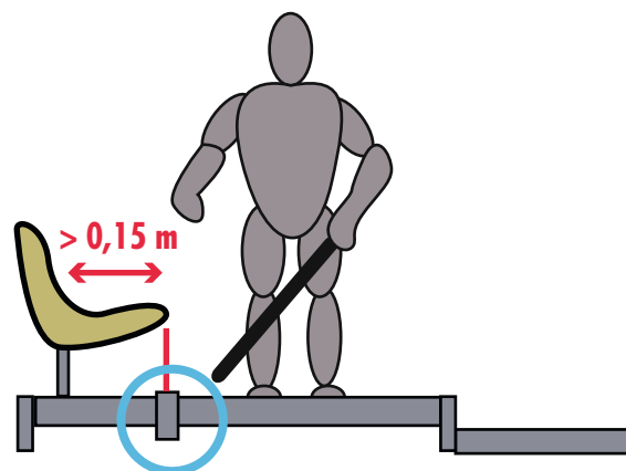
Bordure détectable 3 cm minimum
