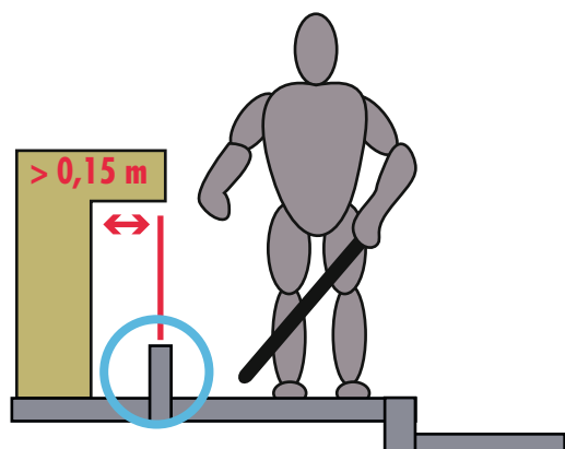
Élément bas détectable 0,30/0,40 m haut
